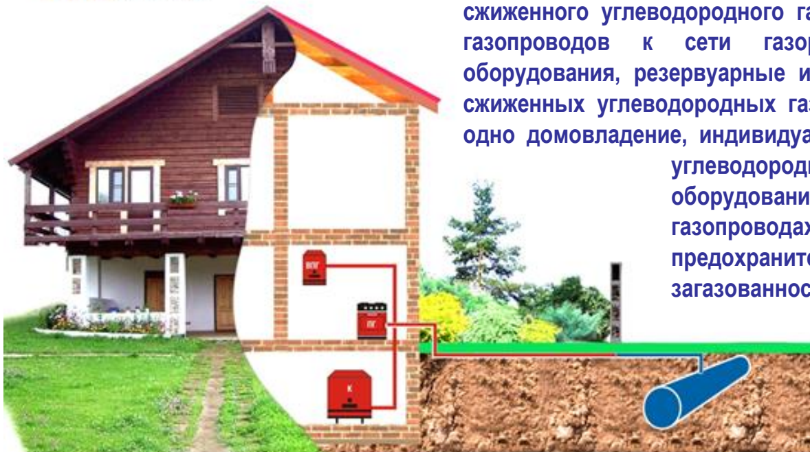
Схема разделения сетей газораспределительной организации и ВДГО домовладения
